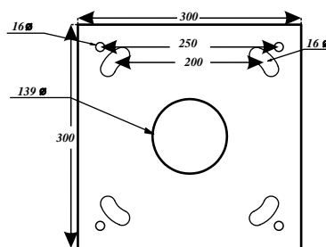
Platine d'ancrage
